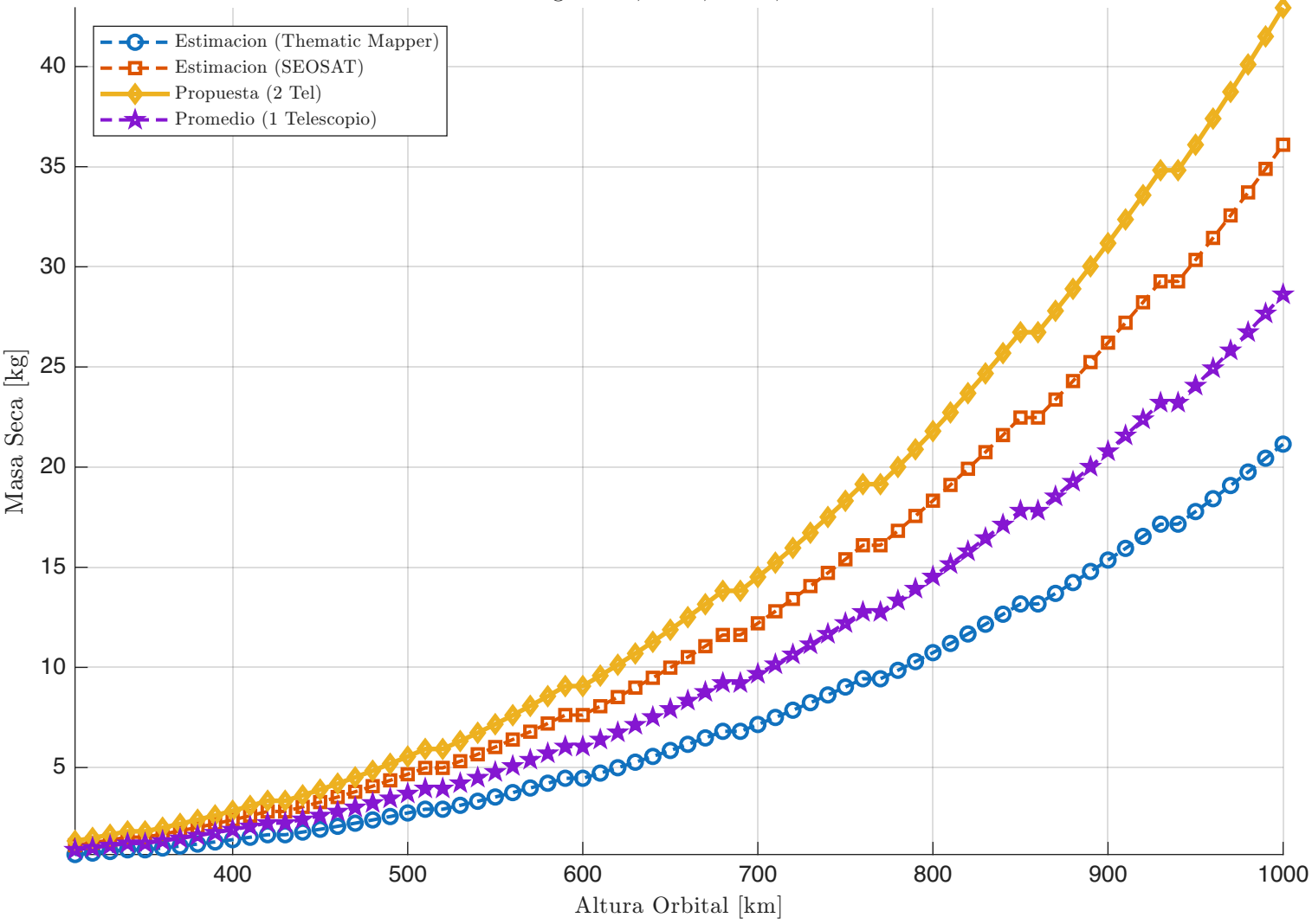
Comparativa de Masa Seca vs. Altura Config: 2 Sat, 2 Tel, Det 3, Korsch
